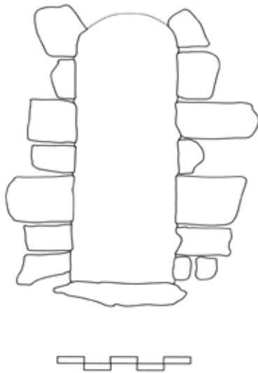
Fig. 27 : porte d'accès à la galerie intra-muros du mur ouest. Relevé G. Auloy, J.-M. Jal, dessin J. V.
