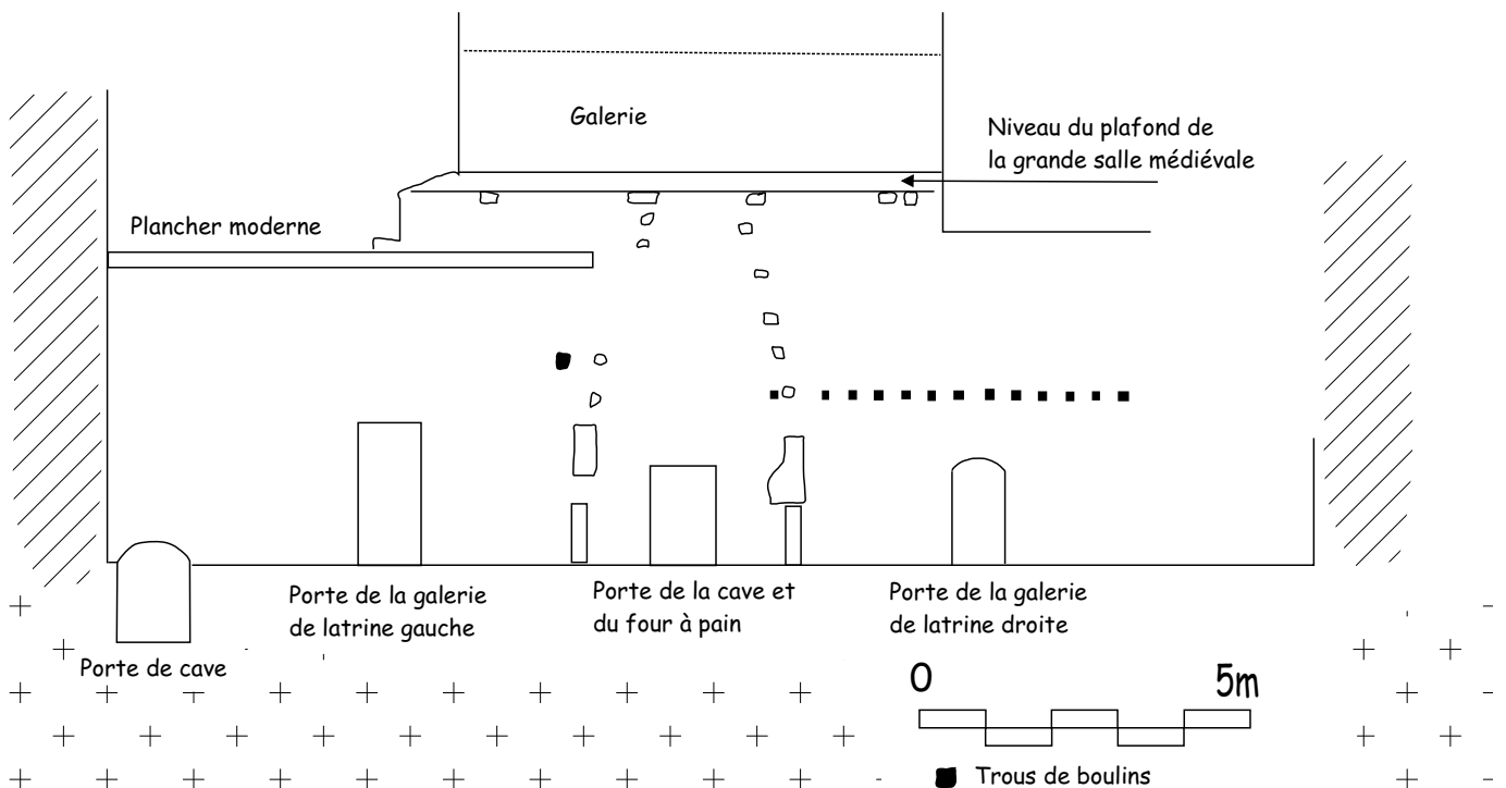
Fig. 18 : mur ouest de la grande salle médiévale. Relevé G. Charleux, dessin J.V.
