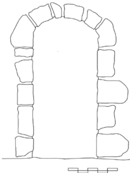
Fig. 13 (ci-dessus) : porte d'accès à la tour ronde depuis le rez-de-chaussée du logis Renaissance. Relevé G. Auloy, J.-M. Jal, dessin J.V.
