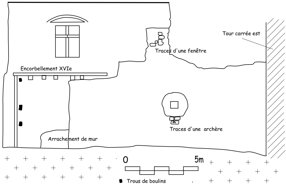
Fig. 6 : courtine orientale, entre l'angle sud-est et la tour carrée est. Relevé G. Charleux, dessin J.V.
