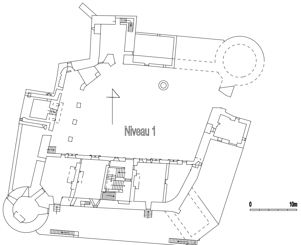
Fig. 3 : plan du château au niveau de la cour ; dessin J. V.
