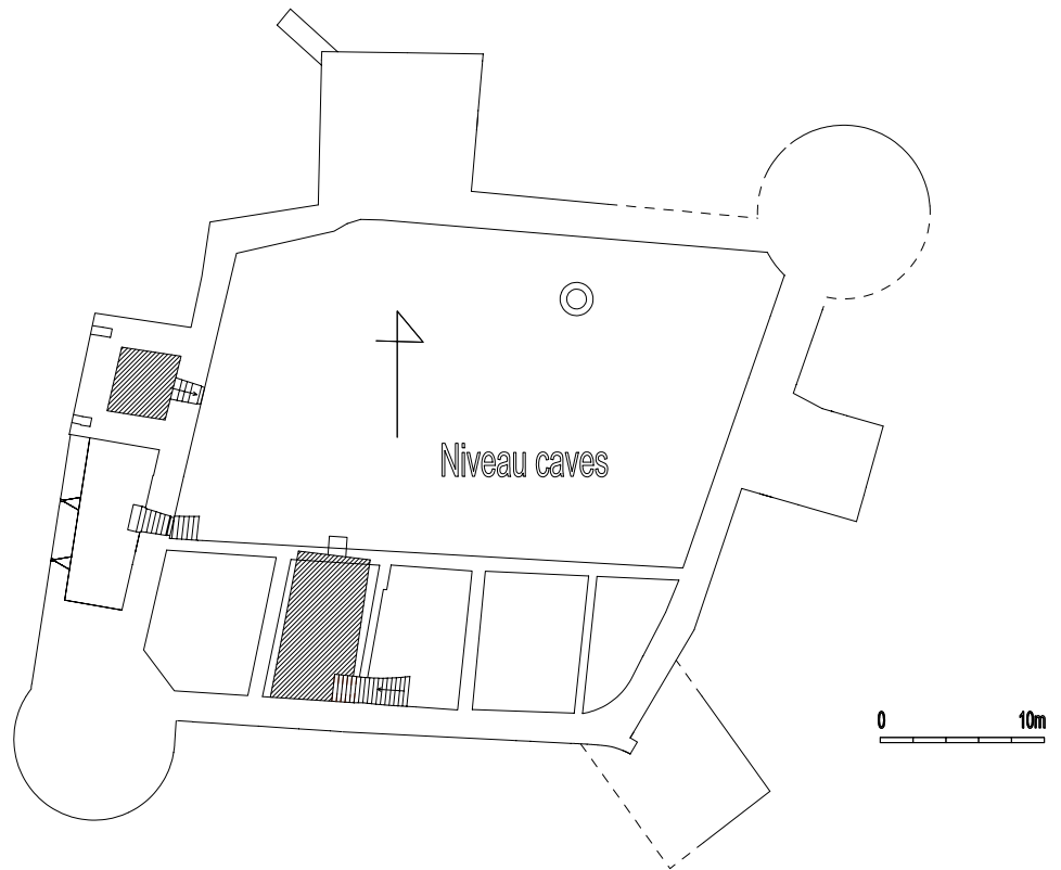
Fig. 2 : plan du château au niveau des caves. Relevé J. Vallet, Br. Colas et G. Auloy ; dessin J. Vallet, CeCaB, 2010.
