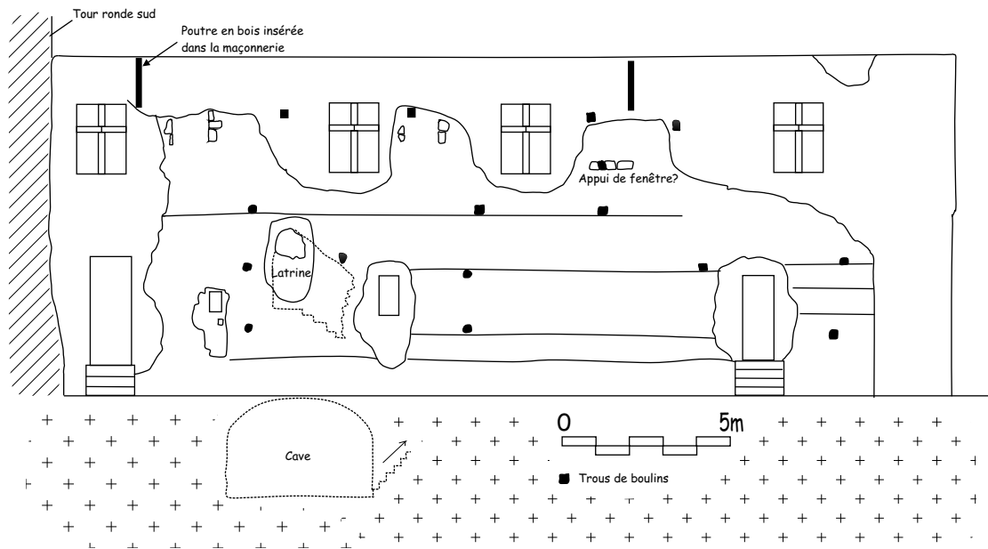
Fig. 9 : courtine sud, entre la tour ronde sud-est et l'angle sud-ouest. Relevé G. Charleux, dessin J.V.
