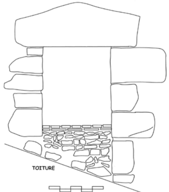
Fig. 28 : porte d'accès à la salle de la tour nord Relevé G. Auloy, J.-M. Jal, dessin J. V.
